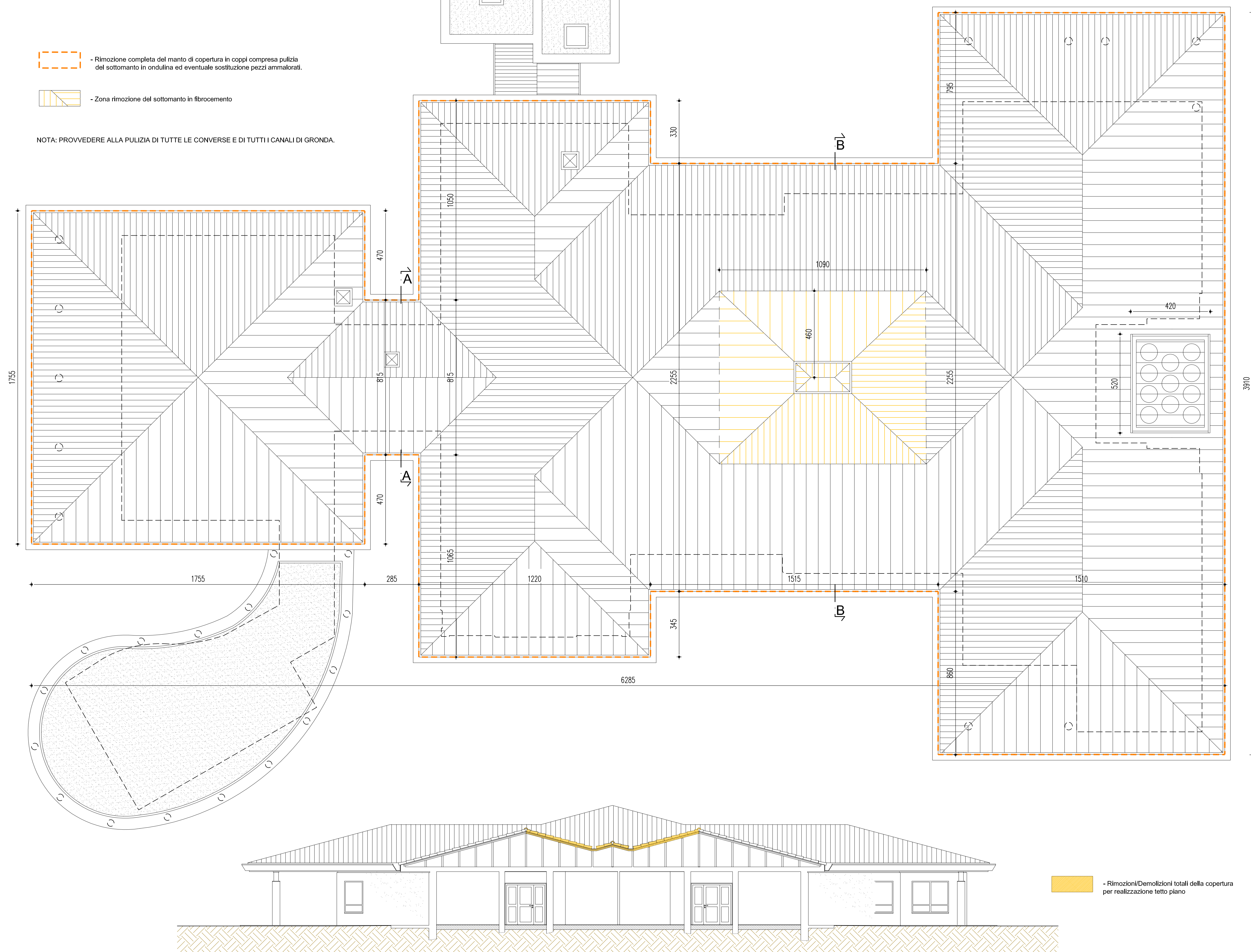
SEZIONE B-B
